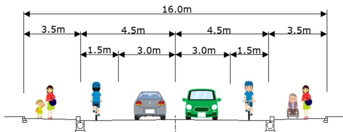
標準横断面図
