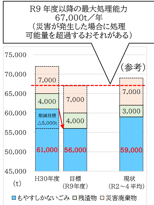
図4. 5,000tの削減目標の根拠
